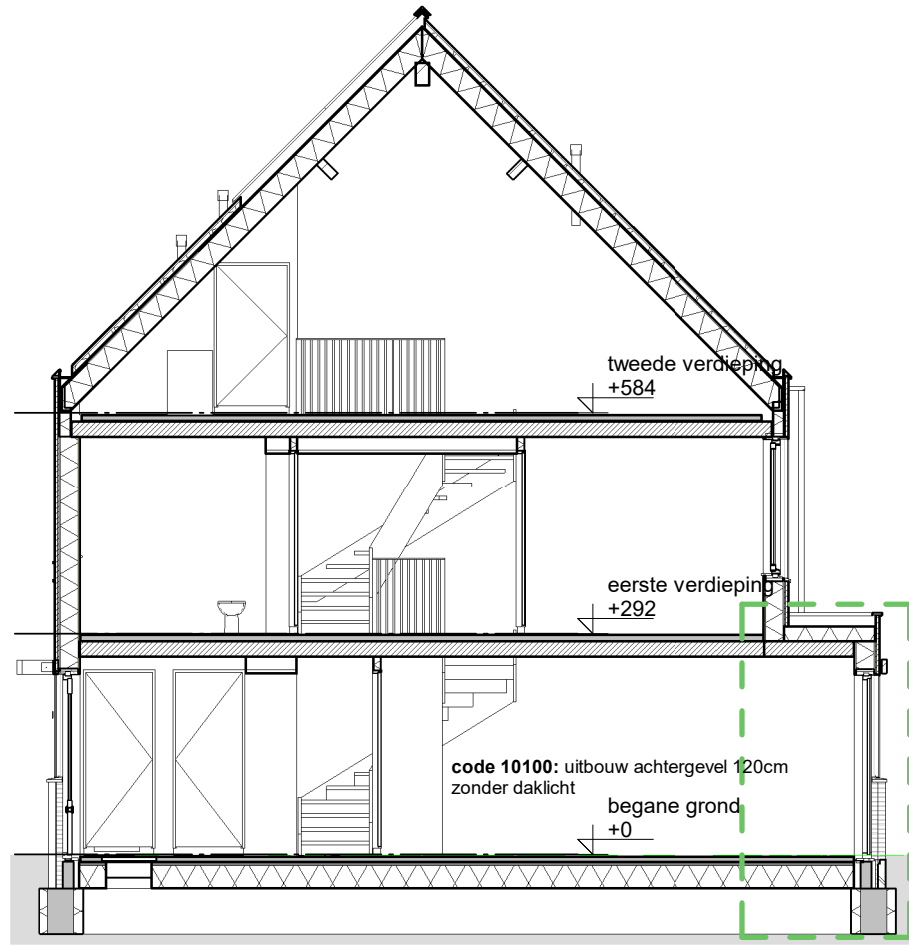
langsdoorsnede
