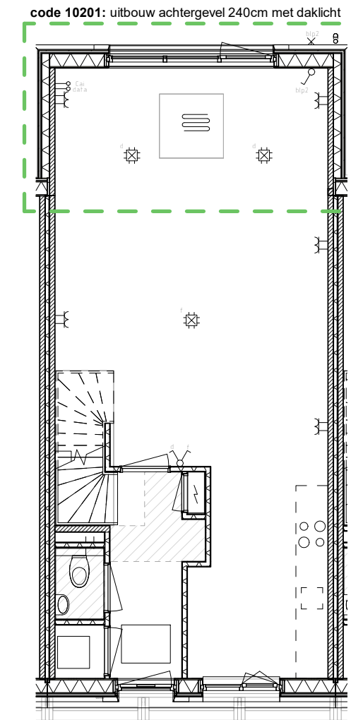
begane grond
