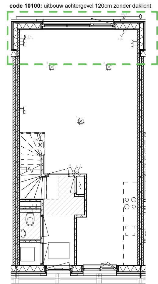
begane grond
