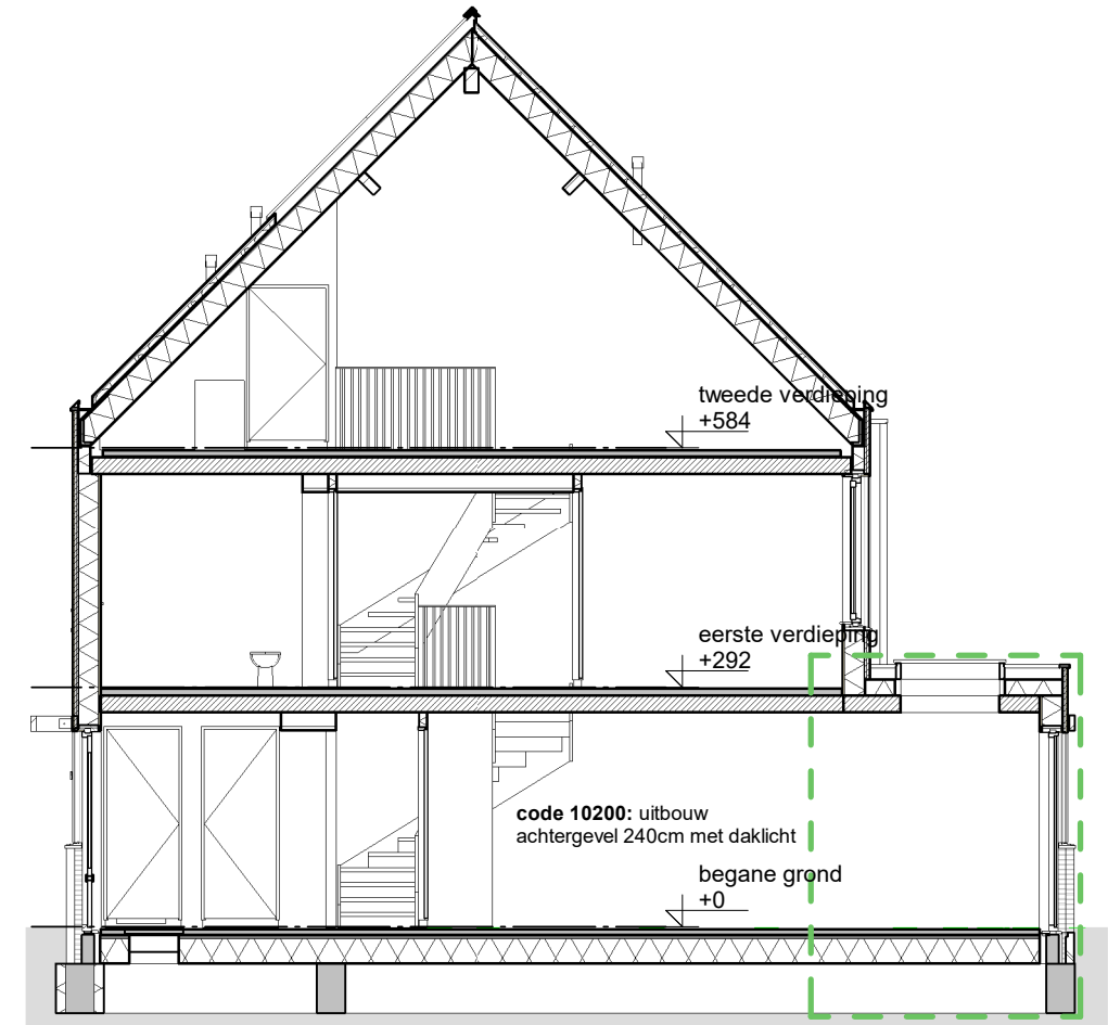
langsdoorsnede
